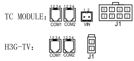
接口管脚示意图:
